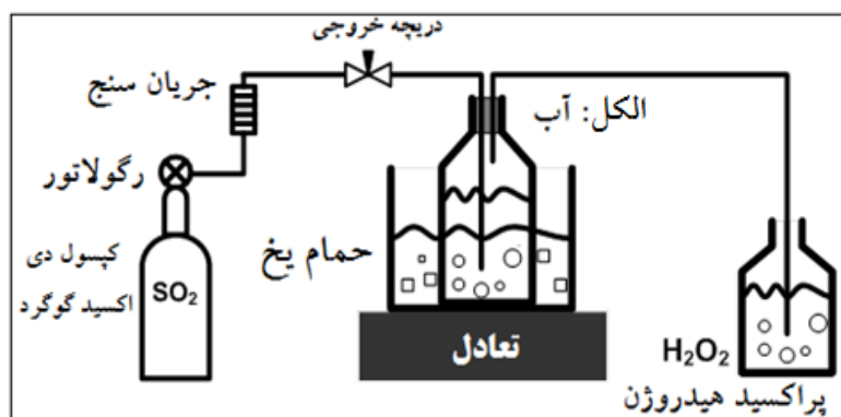
شکل ۱. شماتیک تهیه مایع پخت فرآیند SEW [۱۵].
