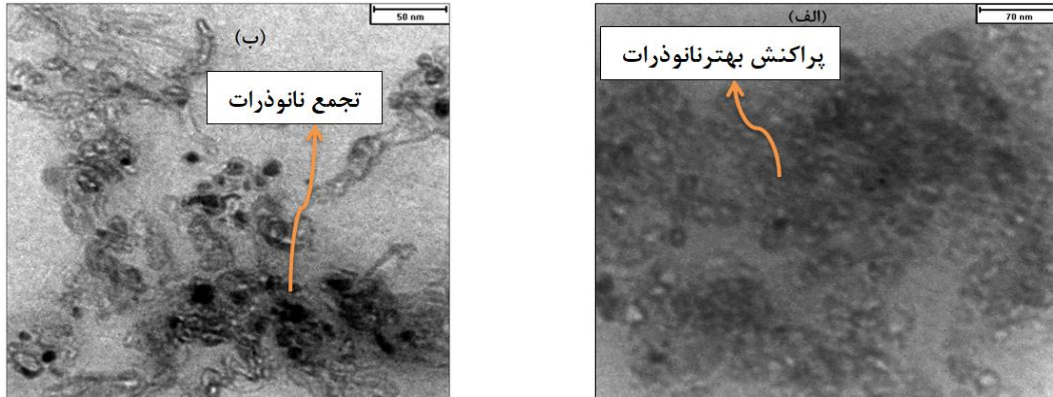
شکل ۷. تصاویر میکروسکوپ الکترونی عبوری (TEM) از فیلم نانوکامپوزیت پلی‌وینیل استات تقویت شده با (الف) ۰/۴ درصد و (ب) ۱/۵ درصد نانوفیبر اصلاح شده
