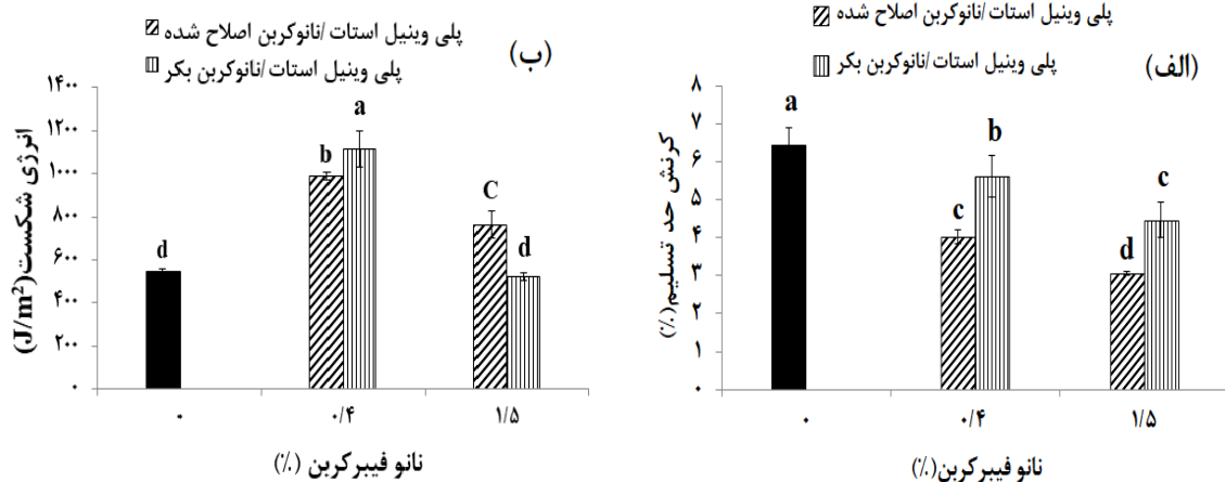
شکل ۶. (الف) کرنش حد تسلیم و (ب) انرژی شکست فیلم نانوکامپوزیت PVAc با نانوفیبر کربن اصلاح‌شده (M) و بکر (V) (حروف انگلیسی متفاوت، اختلاف معنی‌داری را نشان می‌دهد)
