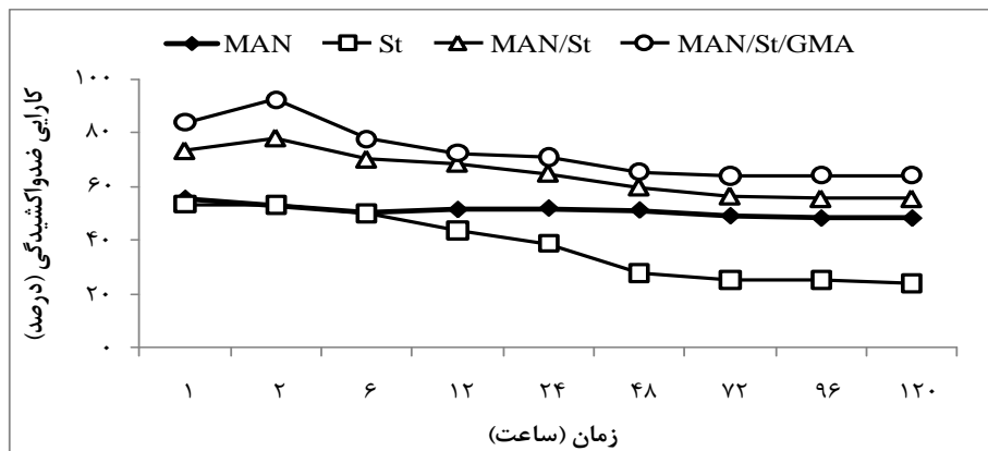
شکل ۷. میانگین کارایی ضد واکنش‌دهی نمونه‌های تیمار شده طی آزمون غوطه‌وری
