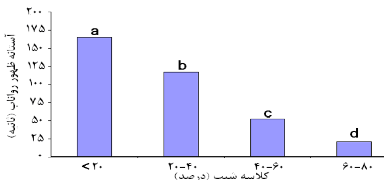
شکل ۷. مقایسه میانگین مقادیر آستانه ظهور رواناب (حروف انگلیسی نام‌شابه نشان‌دهنده معنی‌دار بودن اختلاف میانگین‌ها در سطح احتمال ۵ درصد است)
