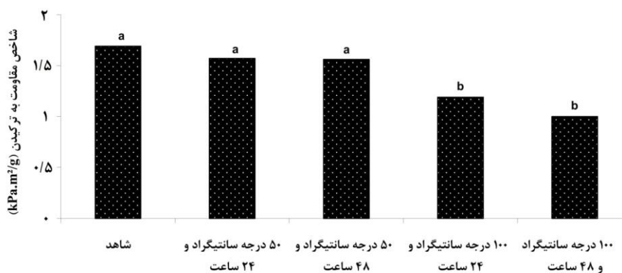
شکل ۲. تأثیر کهنگی تسریع‌شده حرارتی بر شاخص مقاومت به ترکیدن کاغذ
