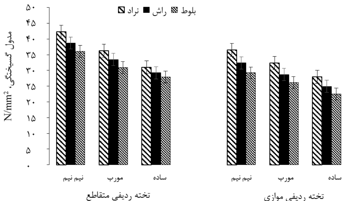
شکل ۴. اثر متقابل نوع اتصال و نوع گونه چوبی بر مدرول گسیختگی (MOR)
