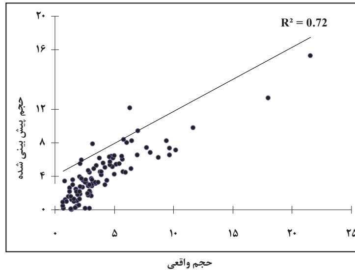
شکل ۱۳. مقایسه خروجی حجم تنه واقعی با خروجی حجم تنه پیش بینی شده توسط مدل دوم جدول ۵
